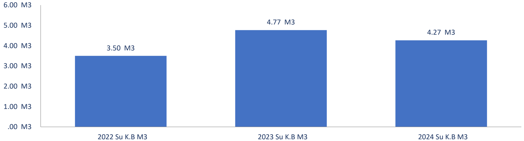
Yıllara Göre Su Tüketim Karşılaştırması (kişibaşı-m3)
