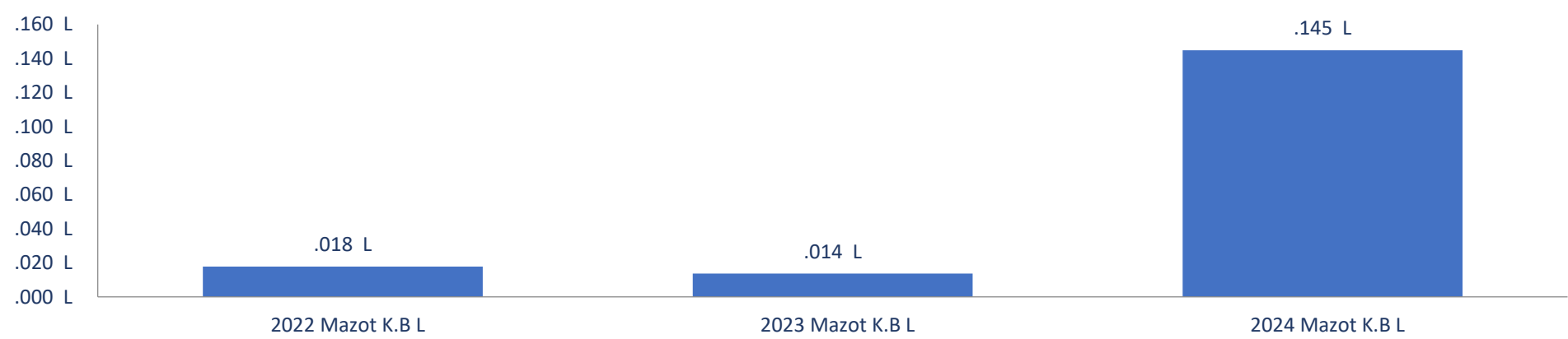
Yıllara Göre Mazot Tüketim Karşılaştırması (kişibaşı - L)
