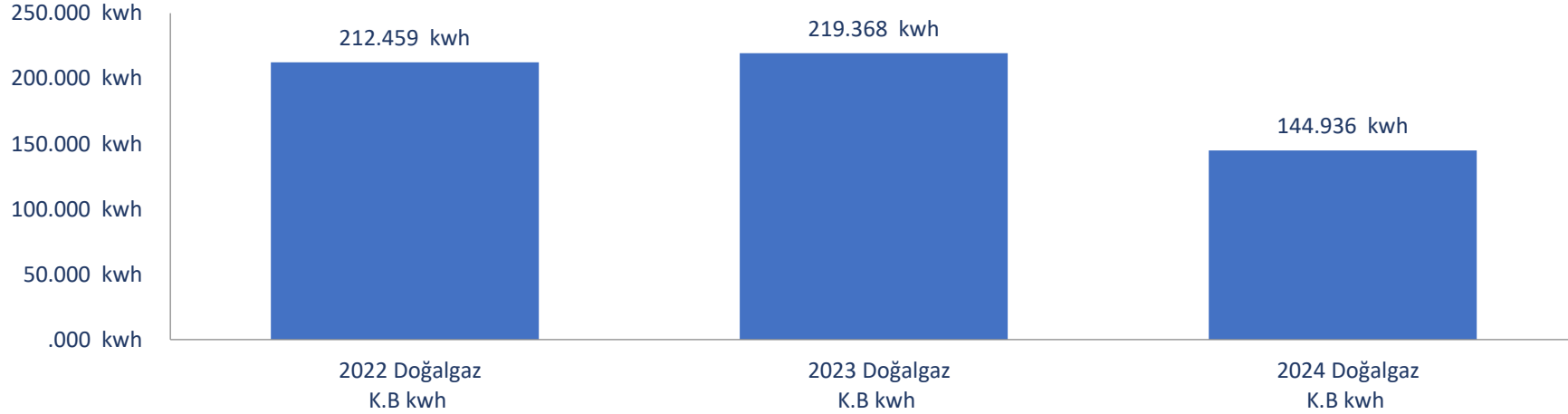
Yıllara Göre Doğalgaz Tüketim Karşılaştırması (kişibaşı - mwh)
